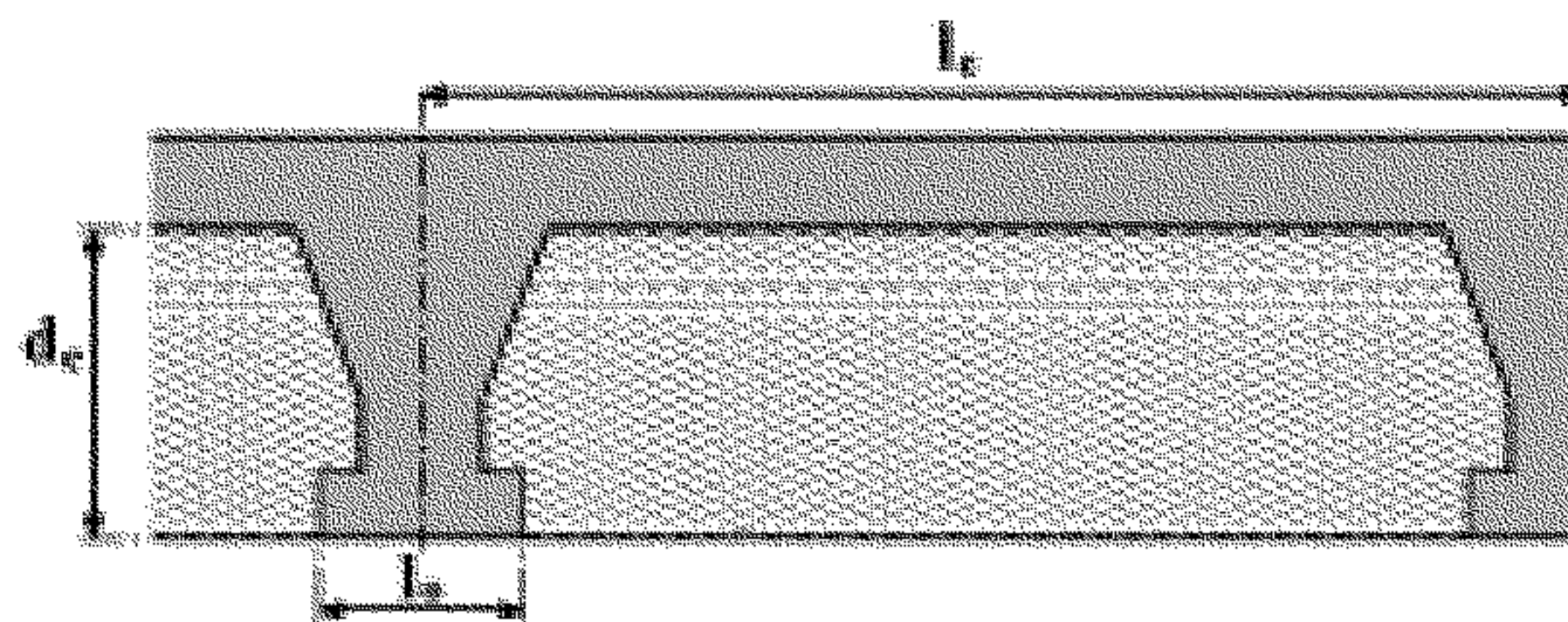
شکل ۶- تیرچه و بلوک پلی‌استایرن ساده
