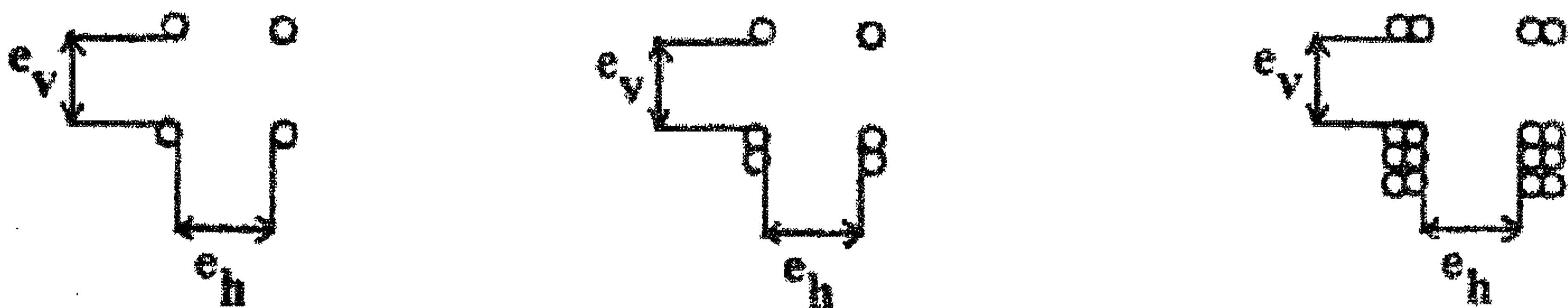
شکل ۲-۲۴-۹ دسته کردن کابل
