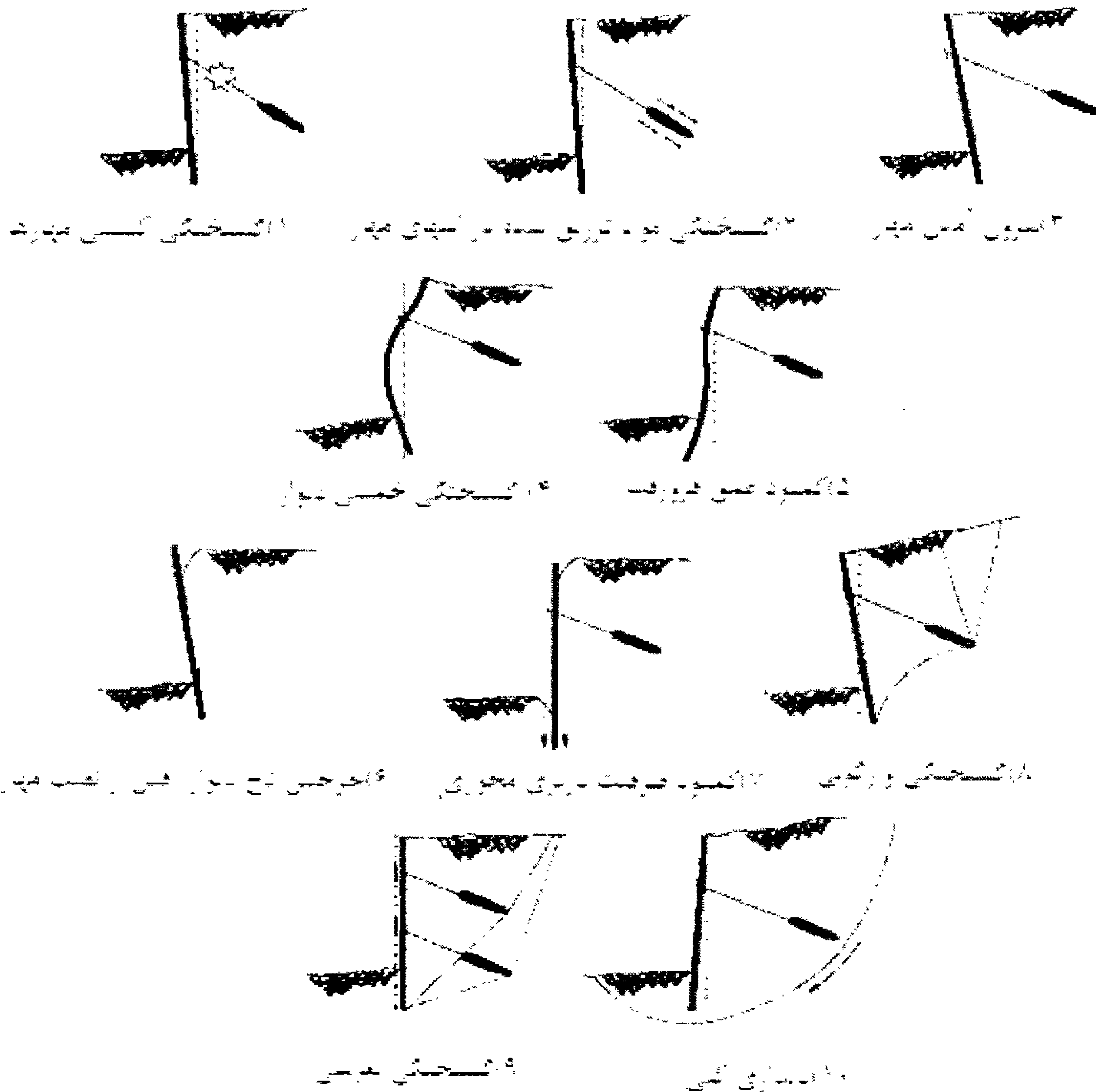
شکل ۷-۵-۱ حالت‌های حدی دیوارهای مهار شده
